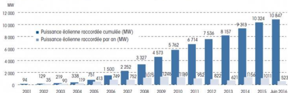
Evolution de la puissance éolienne raccordée cumulée par an (MW)
