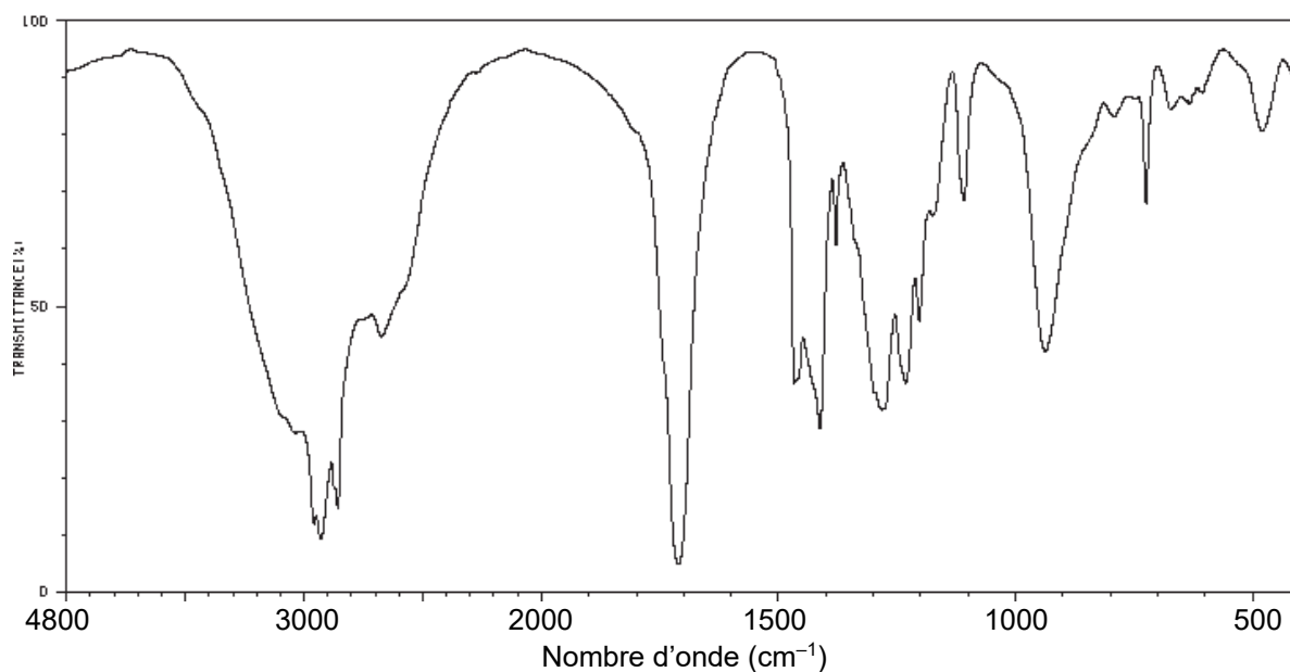
Figure 2. Spectre IR du produit obtenu par sonochimie
