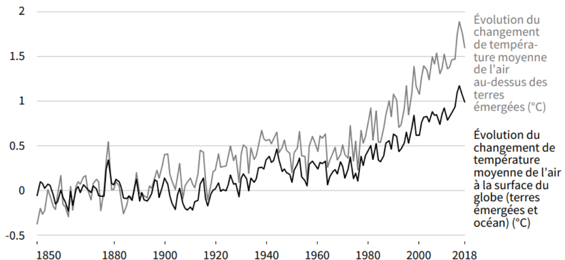
ÉVOLUTION du changement de température par rapport à 1850-1900 (°C)
