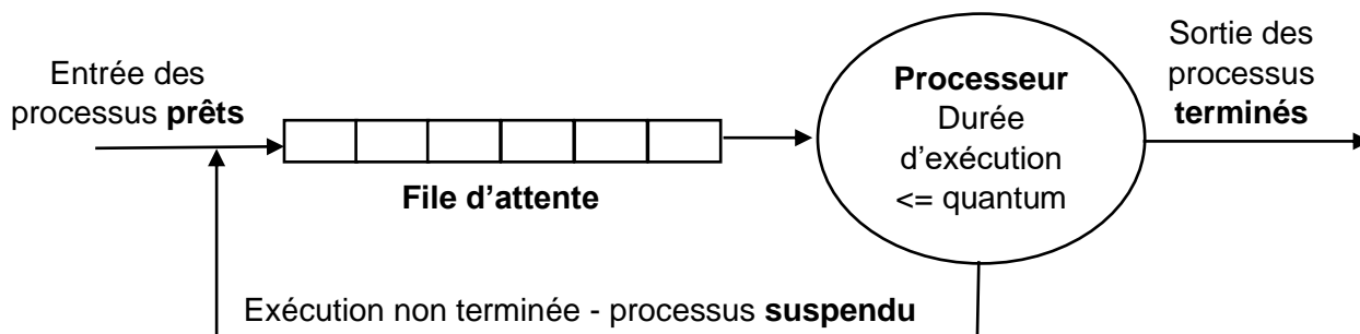
Schéma d'ordonnement du tourniquet
