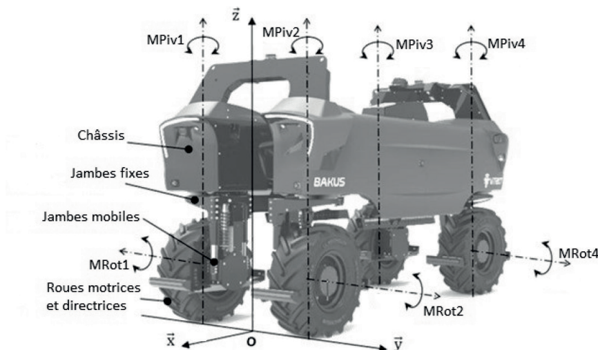
Figure 11 : principaux composants et repère du système étudié
