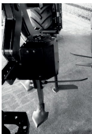
Figure 2 : outils latéraux interceps
