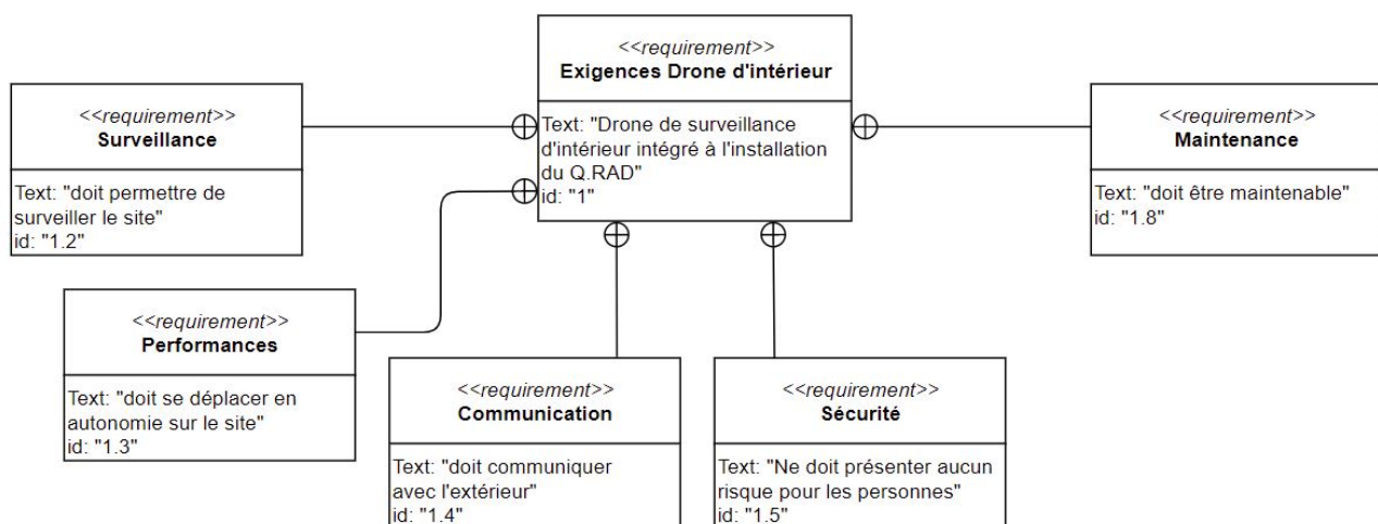
Diagramme des exigences du drone d'intérieur
