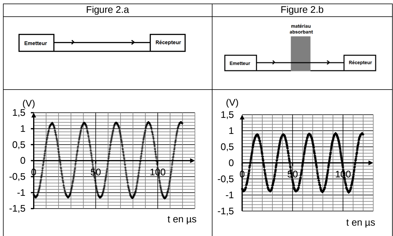
Figure 2 – Étude d'une plaque d'isolant acoustique
