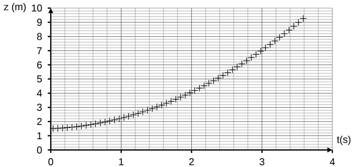
Document 1 – Évolution de l'altitude z du drone en fonction du temps
