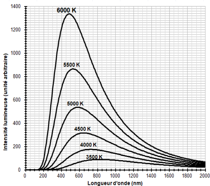
Figure 1a : spectres d'émission du corps noir à différentes températures (exprimées en K).
