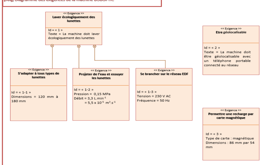
[req] Diagramme des exigences de la machine BOBOPTIC
